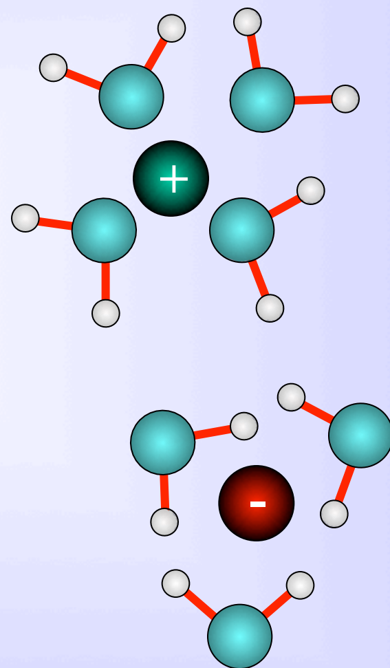
IONI SOLVATATI
